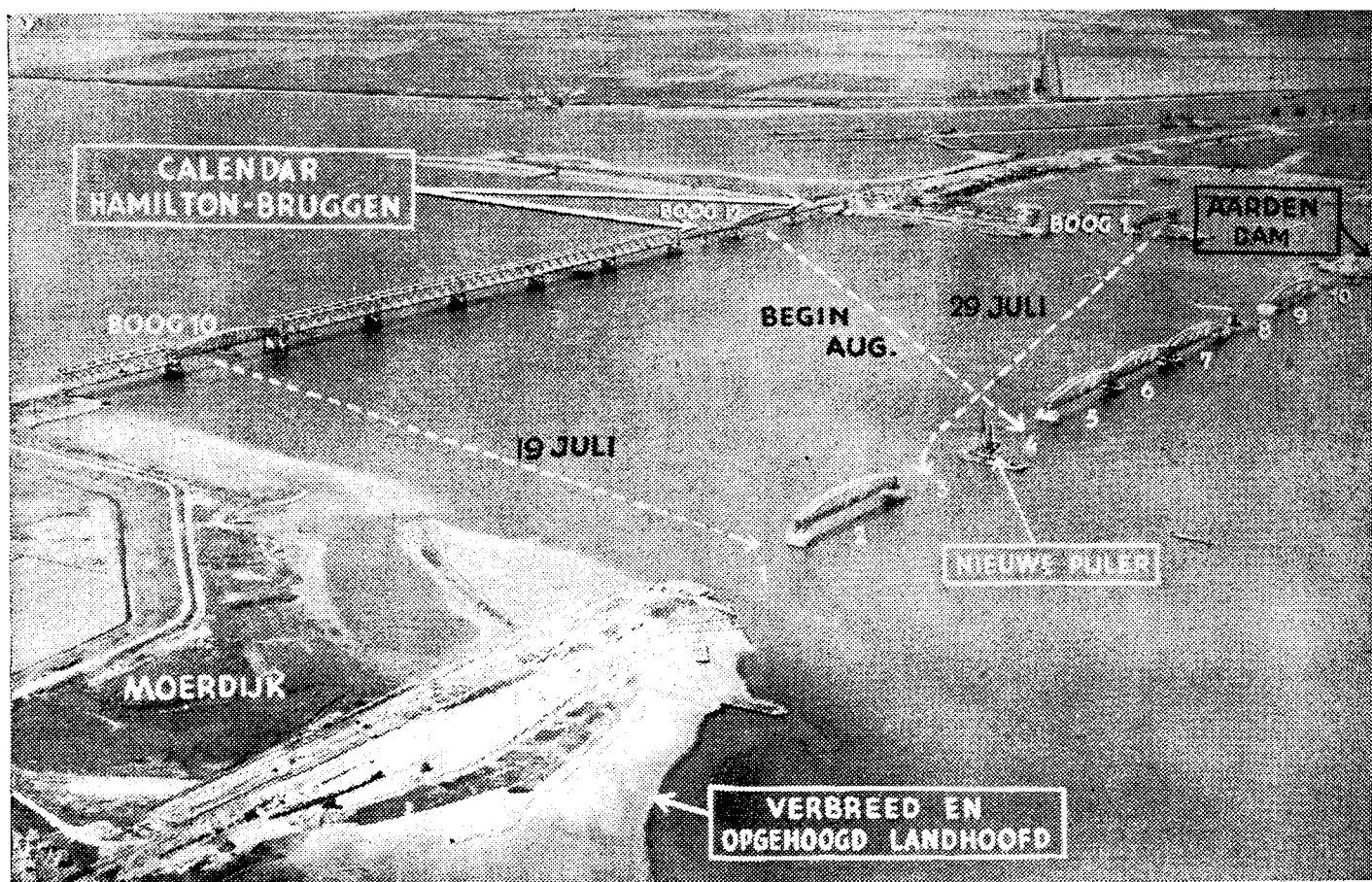
Een overzicht van de werkzaamheden bij den Moerdijk, waar, naar het zich laat aanzien, tegen het eind van deze maand de spoorwegverbinding zal zijn hersteld. Men mist aan de spoor brug thans nog één boog. Wat de verkeersbrug betreft, moet gewacht worden op nieuw materiaal uit Amerika, om de laatste nog aanwezige hulpbruggen door definitieve te vervangen. Tot zoo lang zal men zich met één-richtingsverkeer moeten behelpen.
