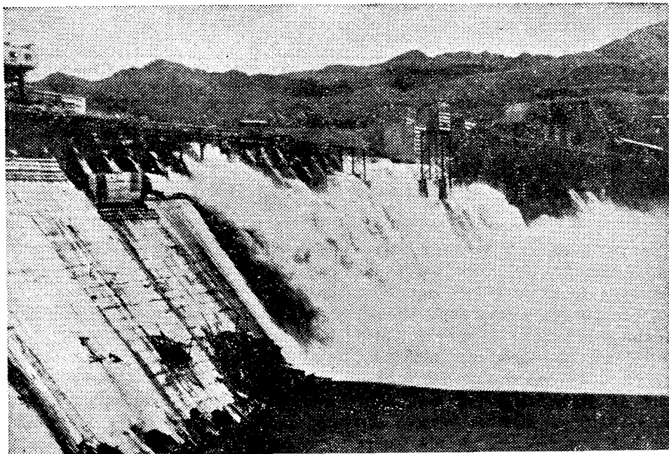
De Japanners hebben de industrialisatie van Mandsjoerijen krachtig bevorderd. De foto toont een stuwdam met electriciteitscentrales.
