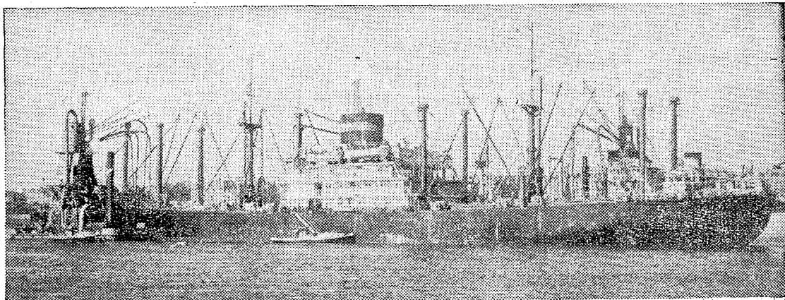
De Friesland in de Rotterdamse Rijnhaven. Een beeld, dat weer hoop geeft voor onze koopvaardijvloot. De Friesland werd in Amerika gebouwd volgens de modernste inzichten.
