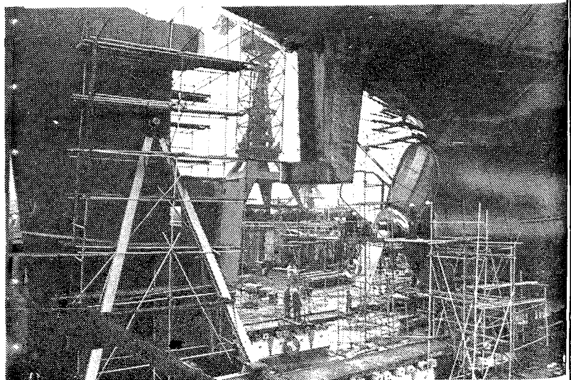
Ruim tien jaar geleden werd nog de ene mammoettanker na de andere gebouwd op de VDSM-werf te Rozenburg. Op de foto een overzicht van de in aanbouw zijnde Esso-Cambria in 1969.
