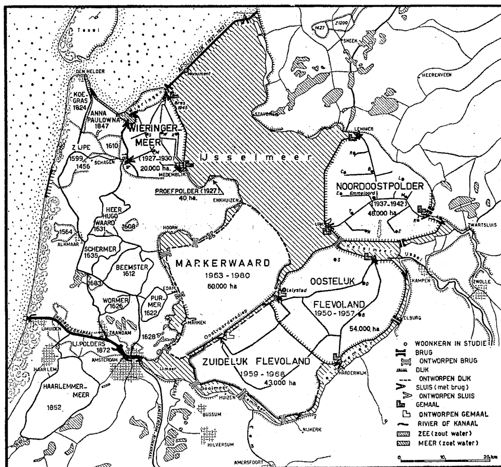
Het Zuiderzeeplan dat thans wordt uitgevoerd.
