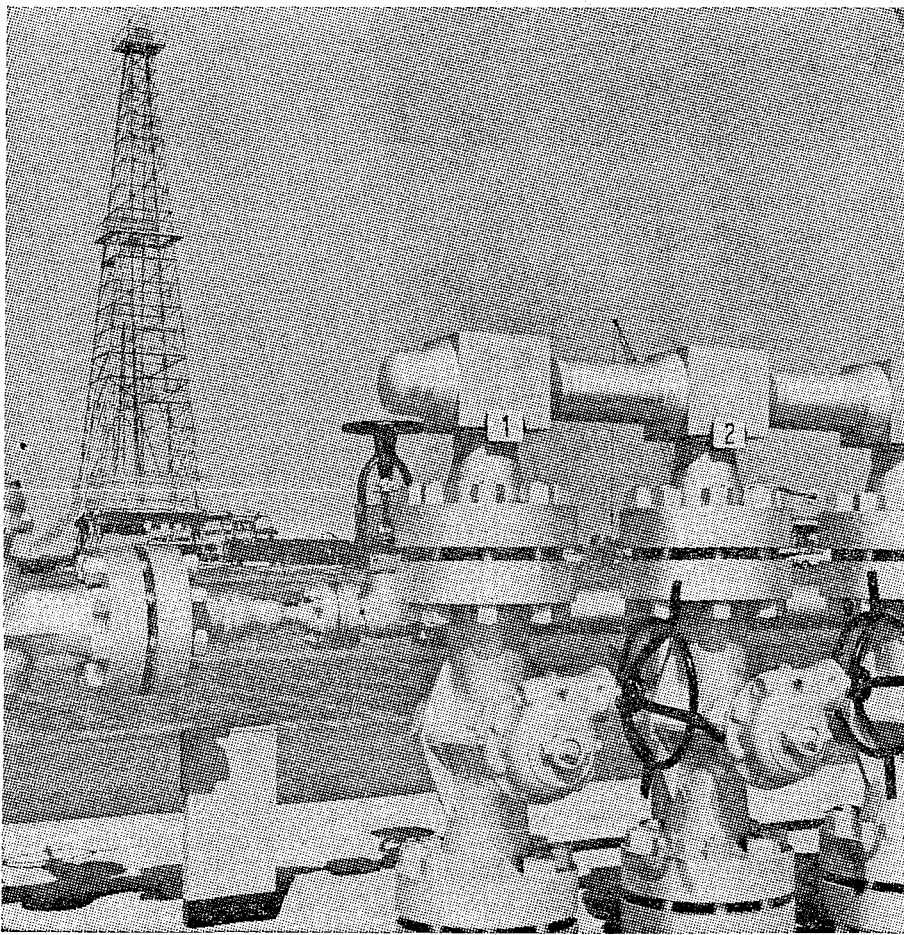
Een deel van het gasveld Slochteren. Op de voorgrond een deel van het zgn. verdeelstuk, waar het gas afzonderlijk kan worden getest.
