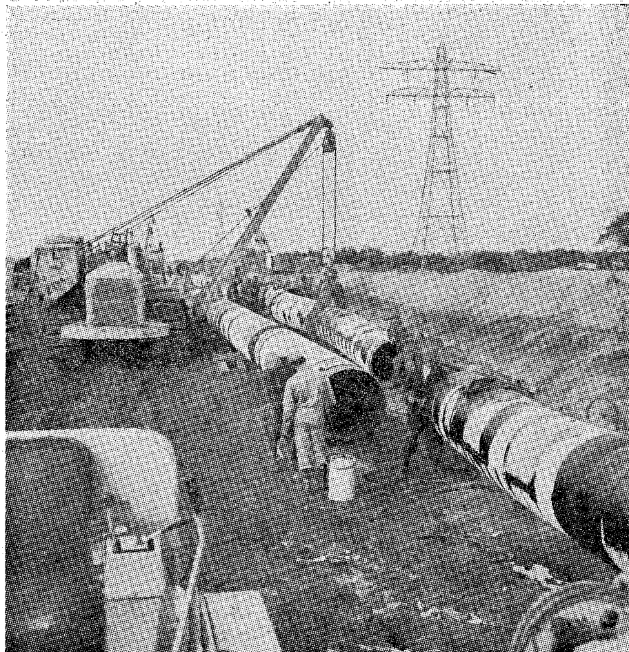
Het leggen van een aardgaspijpleiding in de omgeving van Zuidwolde (Dr.).
