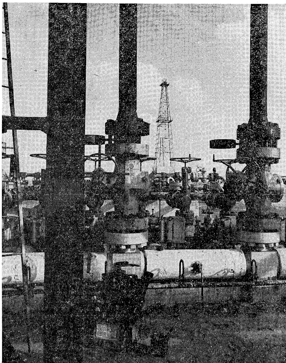
Een overzicht tijdens de bouw van de gasdrooginstallatie op het aardgasveld Slochteren. (N.A.M.-foto)
