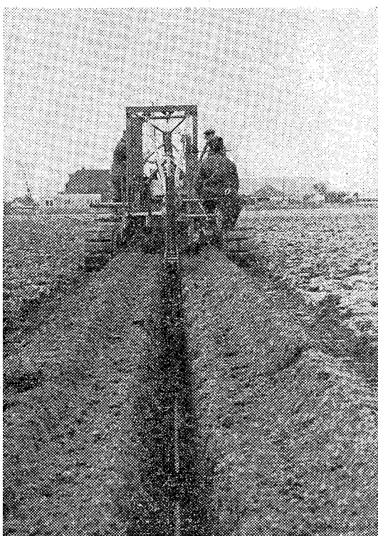
Een draineer-machine, die niet alleen de draineersleuf graaft, doch tegelijk de draineerbuizen — hier plasticbuizen — legt.
