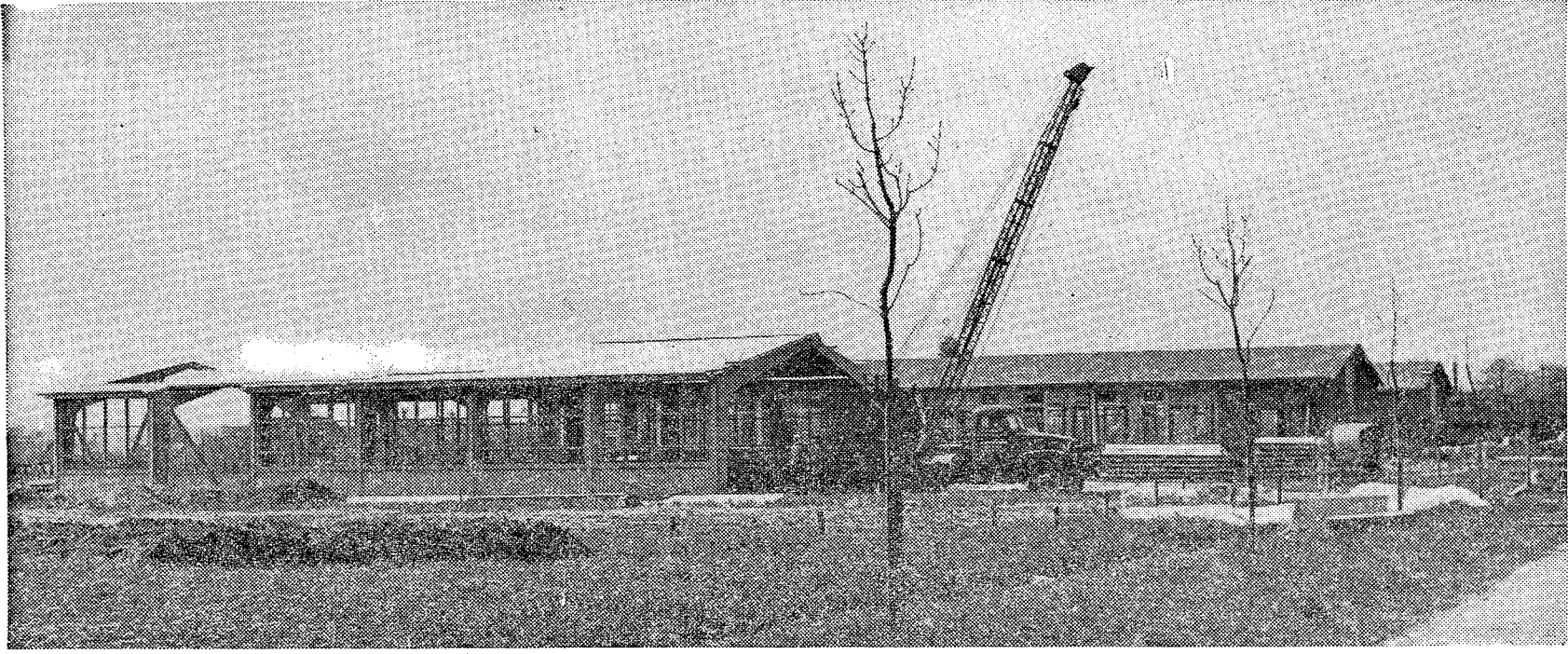
Bovenstaande foto geeft een beeld van de montage van enkele hallen bestemd voor de - tijdelijke - onderbrenging van de Philipsindustrie te Stadskanaal.
