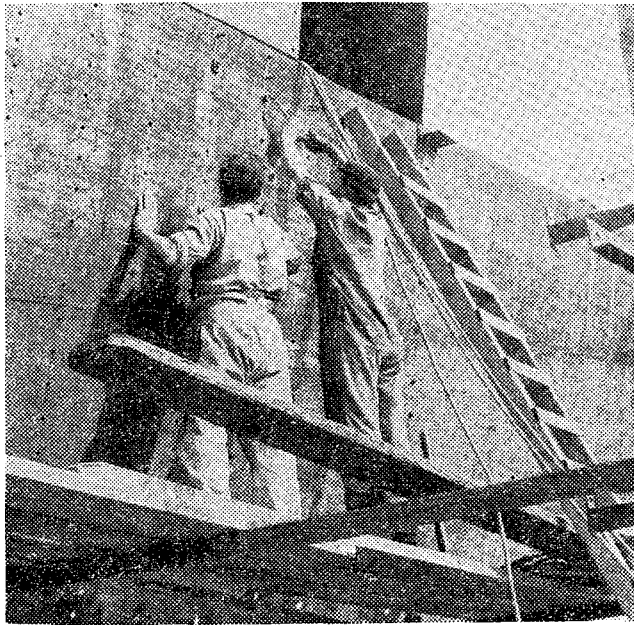
Ook op de middelgrote werven wordt steeds meer sectie-bouw toegepast. De in de loods gelaste secties worden na veel manoeuvreren vakkundig op de juiste plaats gevoegd.
