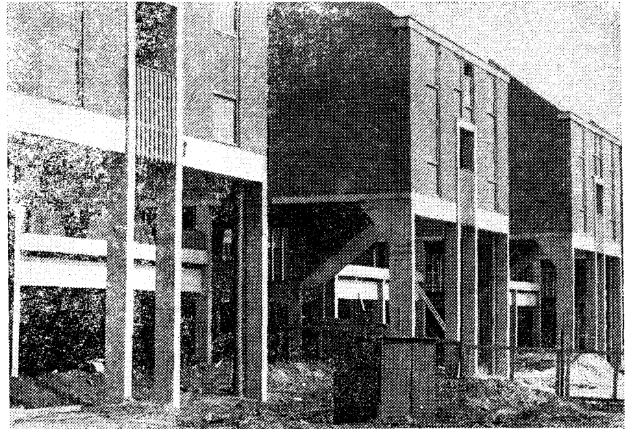
Een experimenteel bouwplan, door het rijk gesubsidieerd, in de gemeente Hengelo (O.): het Kasbahproject van de architect Pieter Blom. Evenals het plan Zilverkamp in Huissen een gemengde vorm van wonen. De Kasbahhuizen staan alle op palen.
