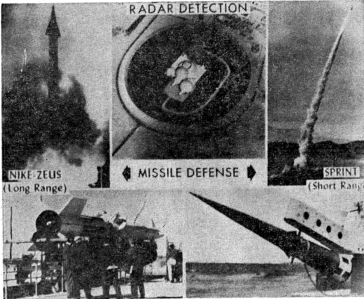
Overzicht van de belangrijkste onderdelen van het „dunne“ Nike-X-raket-afweersysteem, dat de Verenigde Staten tegen eventuele Chinese aanvallen gaan opbouwen. Linksboven en beneden de lange afstand Zeus-raket, geheel rechts de Sprint-raket voor korte afstand en in het midden boven een radarcentrum.
