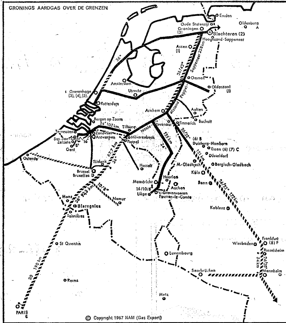
— voltooide hoofdvoedingsleidingen - - - - - geprojecteerde of in aanleg zijnde hoofdvoedingsleidingen
