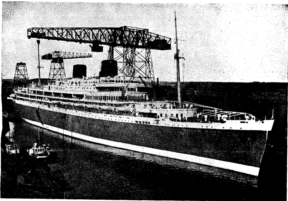
De „Willem Ruys”, het grootste schip, dat „de Schelde” bouwde, ligt klaar om naar z'n bestemming te vertrekken.
