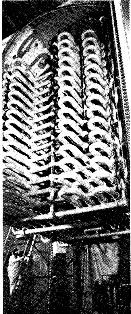
De tanks, waarin het hoogradioactieve afval uit opwerkingsfabrieken in opgeloste toestand wordt bewaard, zijn dubbelwandig. De foto toont het aanbrengen van de koelspiralen in een tank te Windscale, Engeland. Zeven, van elkaar onafhankelijke spiralen moeten de warmte, die bij de radioactieve ontleding vrijkomt, afvoeren.
